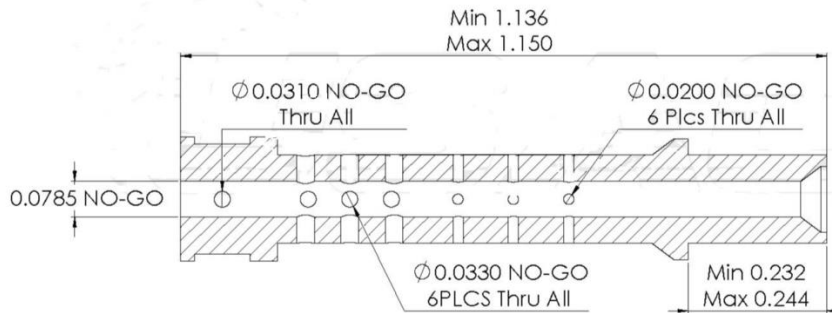
GX 160 UT 2 DUMP TUBE
